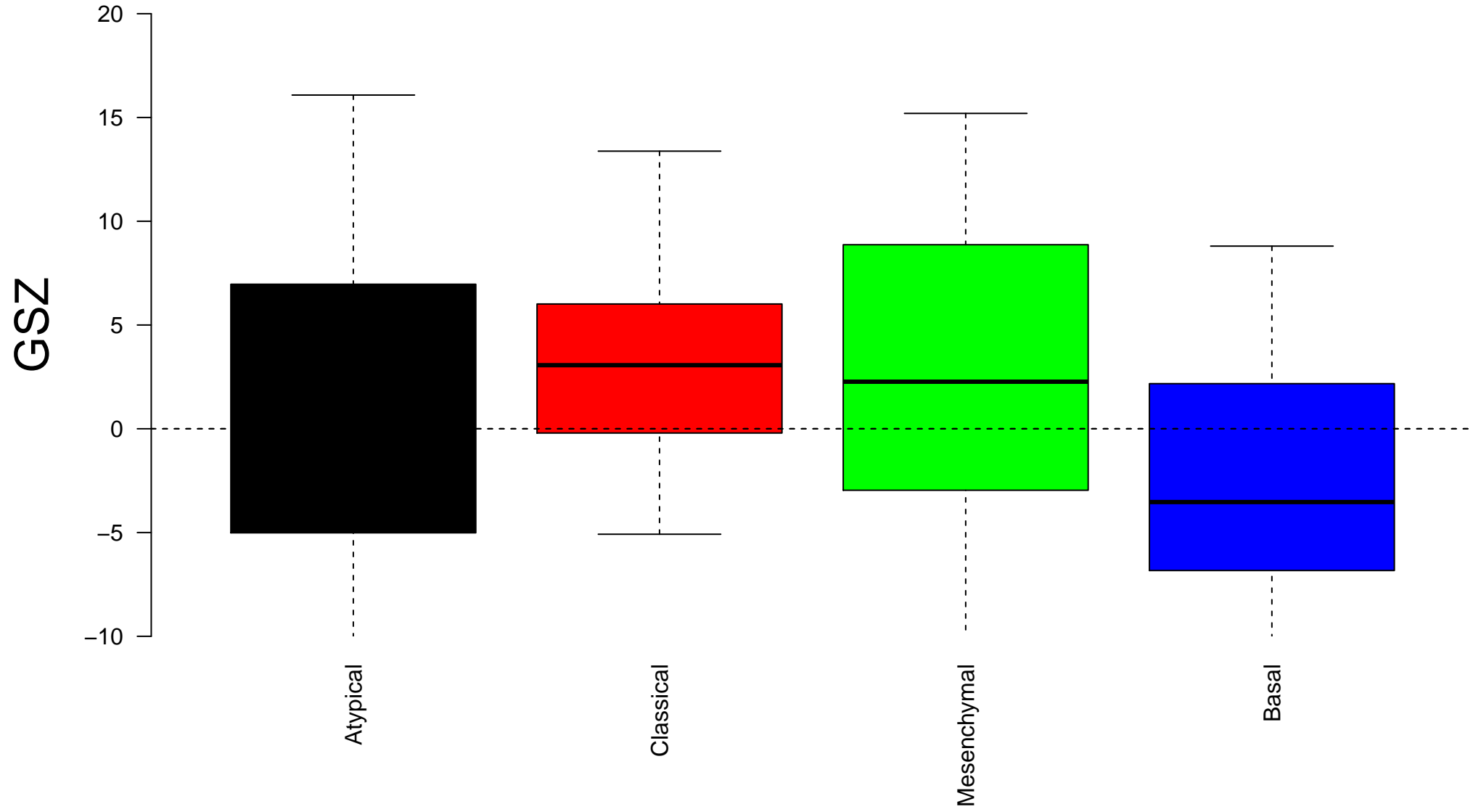
willscher_GBM_Verhaak-PNmut_expression_C_down
